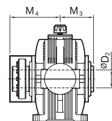
Hollow Output Shaft With Shrink Disk - (D)
