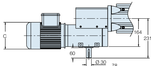
Gearbox with AC motor Getriebe mit Asynchronmotor Réducteur avec moteur asynchrone
