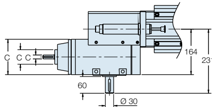
Gearbox with free input shaft Getriebe mit Antriebswelle Réducteur avec arbre nu
