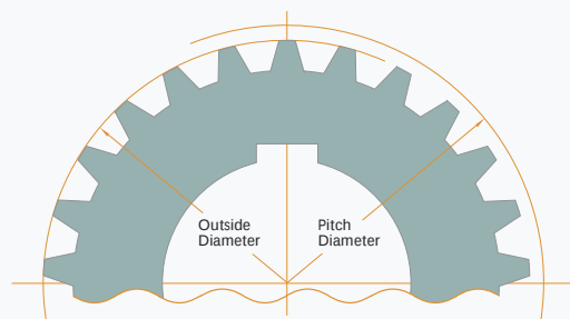
SPROCKET PROFILE
